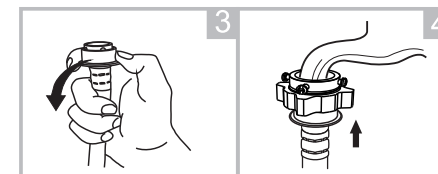
Druk op de schuifring en stop de toevoerslang in de onderkant van het koppelstuk
