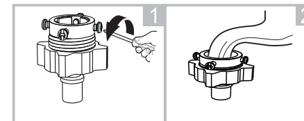
Draai de vrije moer en de vier schroeven los
