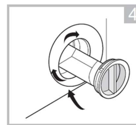
4 Revisser le filtre complètement dans forcer et remettre la trappe
