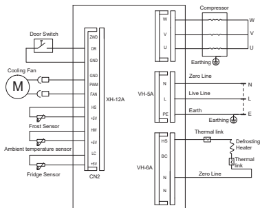
Schéma électrique
