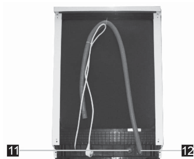
Vue arrière
