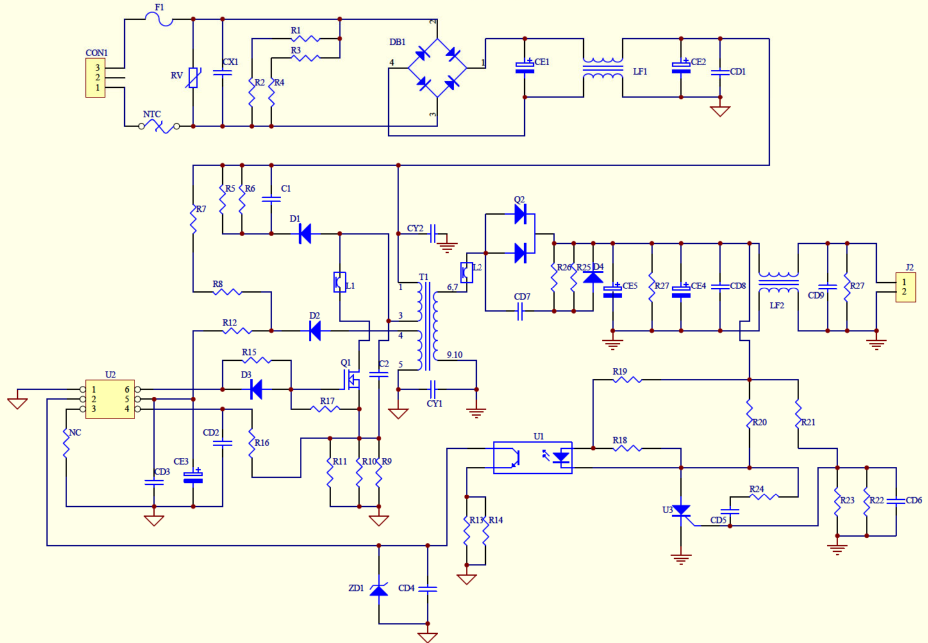
QDPOWER-GF-015030A Ver1.0原理图
