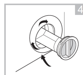
Revisser le filtre complètement dans forcer et remettre la trappe
