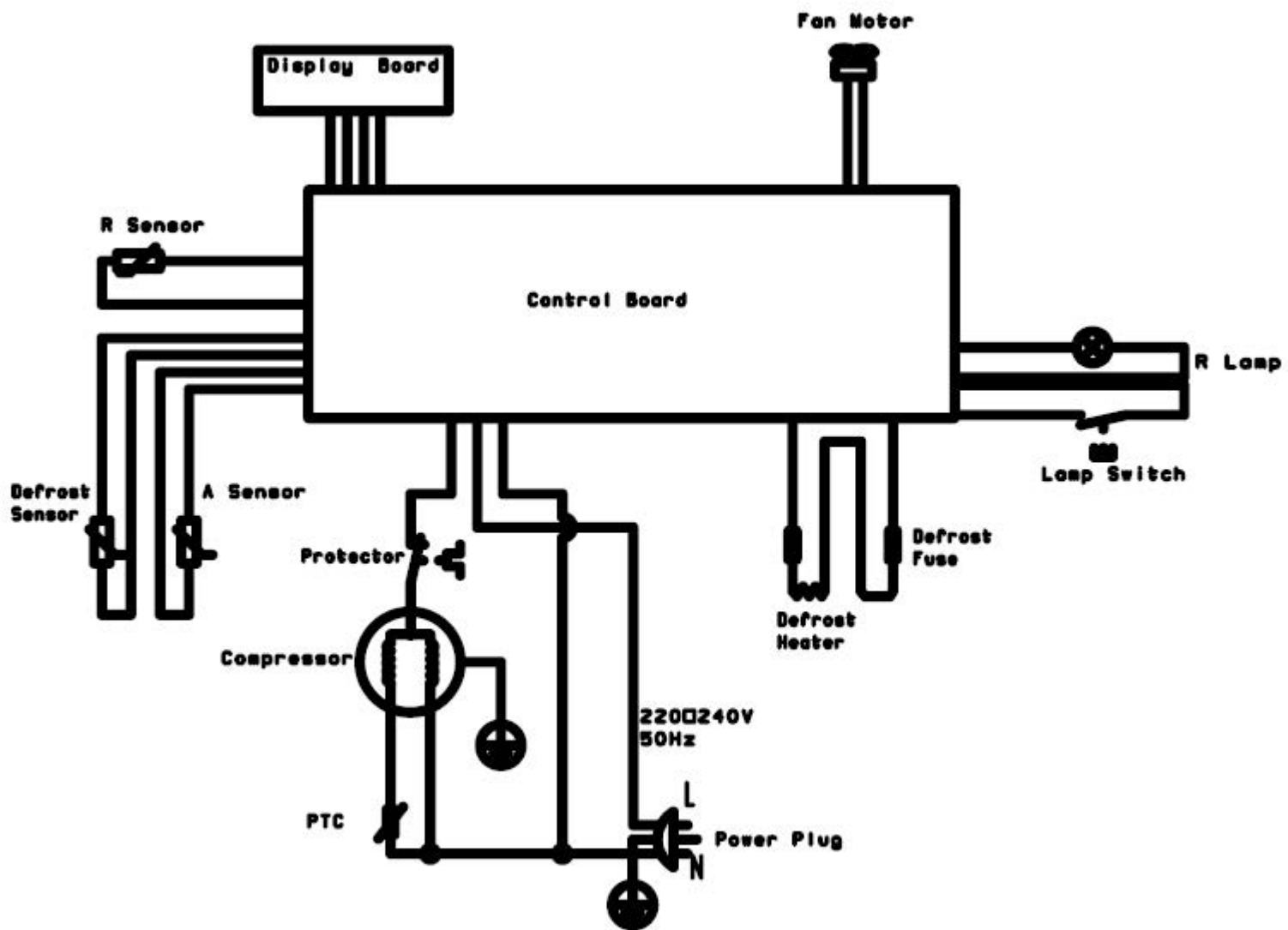
CE-BCD276WE 电路图
