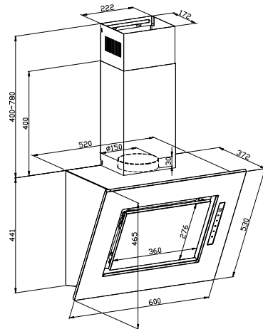
SHD60XPERI/2
