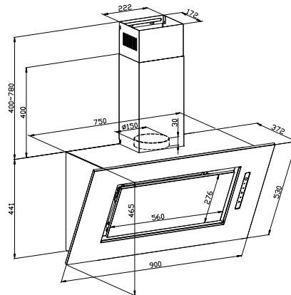
SHD90XPERI/2
