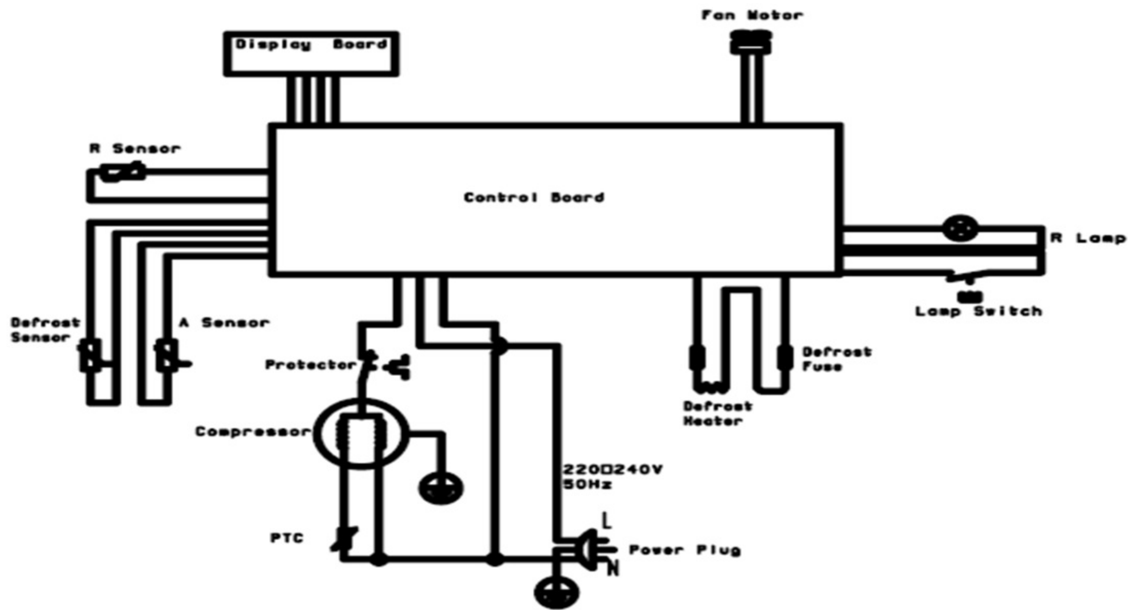
CE - BCD308WE 电路图
