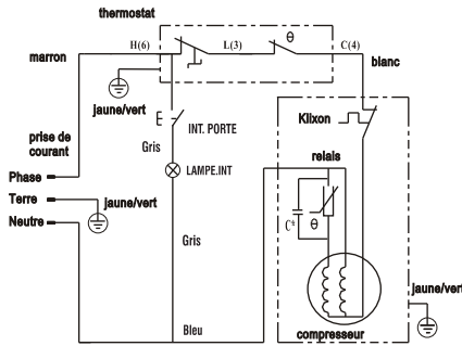
C* Le condensateur est optionnel selon le modèle du compresseur
