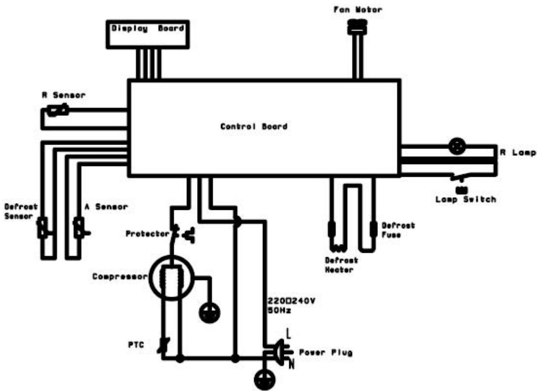
CE-BCD308WE 电路图
