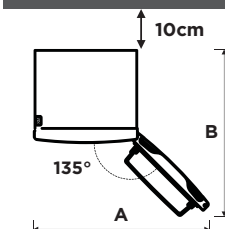
Вигляд згори
