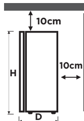
Вигляд збоку
