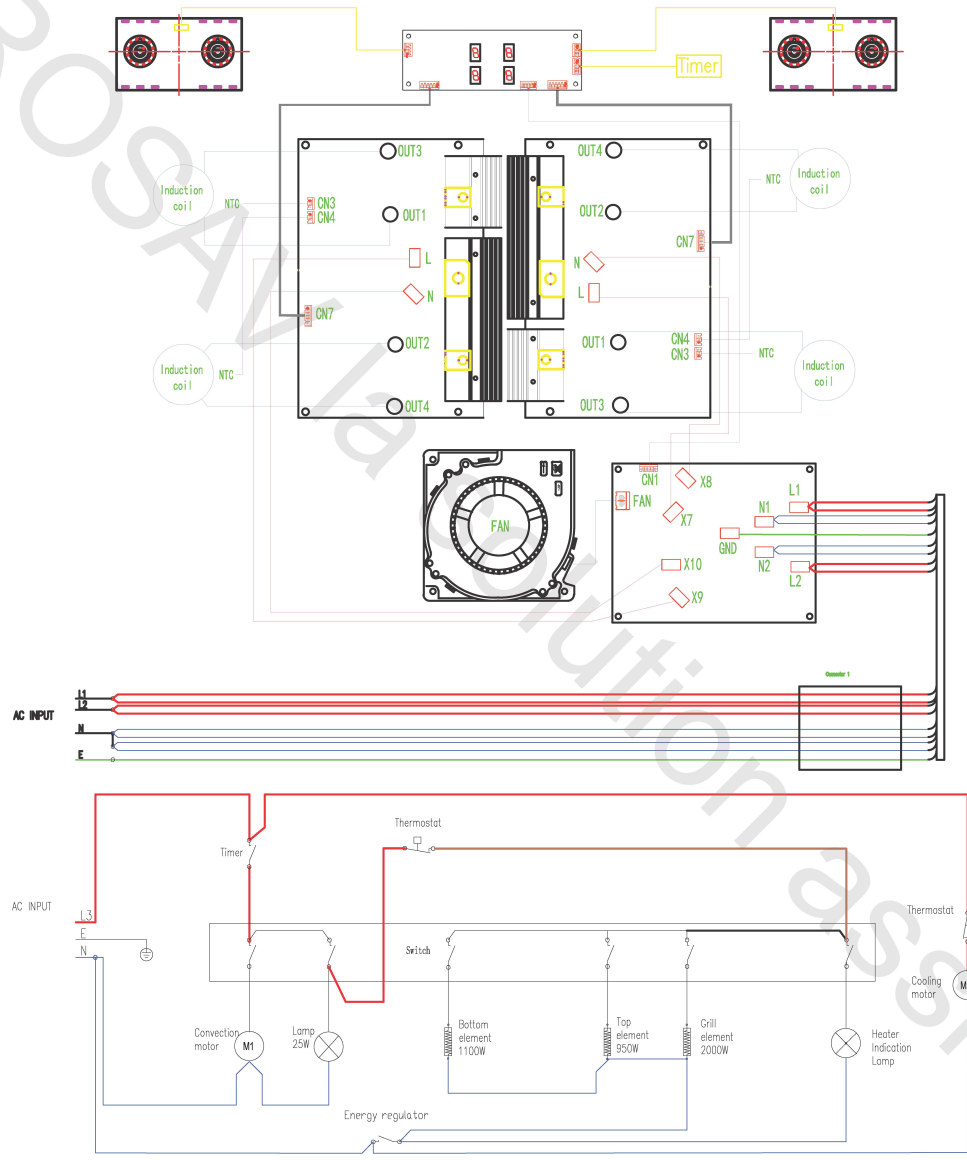
组合炉冷电器原理图
